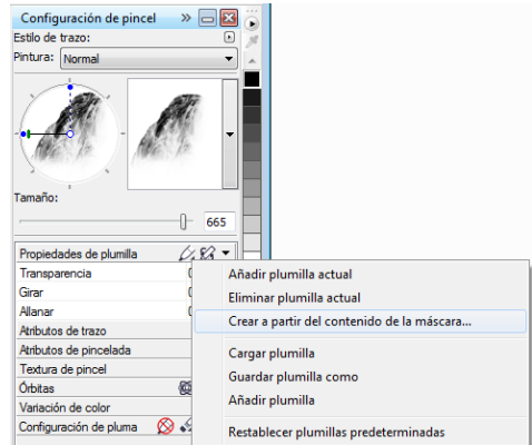
Figura 8: creación de una plumilla de pincel a partir de la máscara
