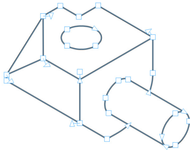
Abb. 64 Ideale Kurvenqualität keine unnötigen doppelten Knoten, Splines statt Polylinien, nur wenige Knoten je Spline
