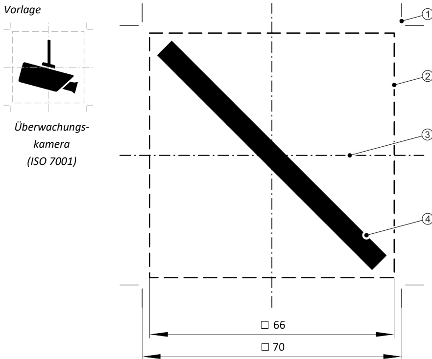
Abb. 51 Vorlage für Symbole nach ISO 22727 [mm]
