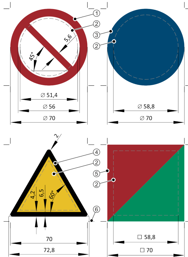
Abb. 52 Formen für Sicherheitszeichen nach ISO 3864 [mm]
