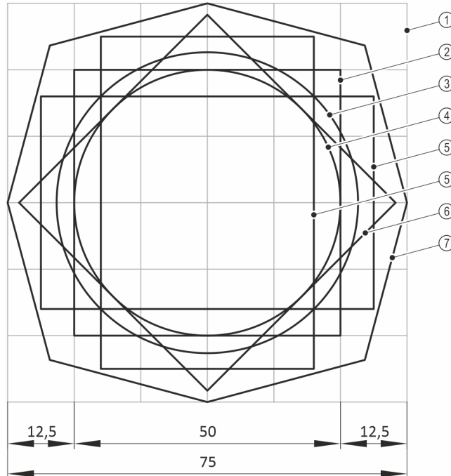
Abb. 53 Grundfigur für Symbole aus ISO 80416 [mm]
