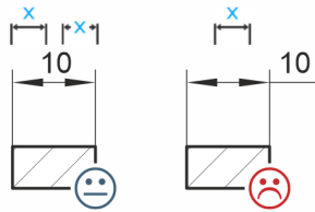
Abb. 42 Probleme beim Bemaßen kleiner Dimensionen
