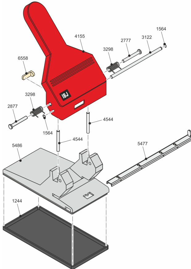
Abb. 61 Locher in einer Explosionsdarstellung
